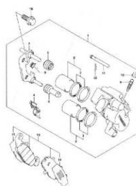
FIG.57 FRONT CALIPER (J-10)
